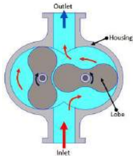
Fig. 5.1.5 Lobe compressor
