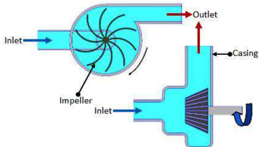
Fig. 5.1.6 Blower (Centrifugal type)
