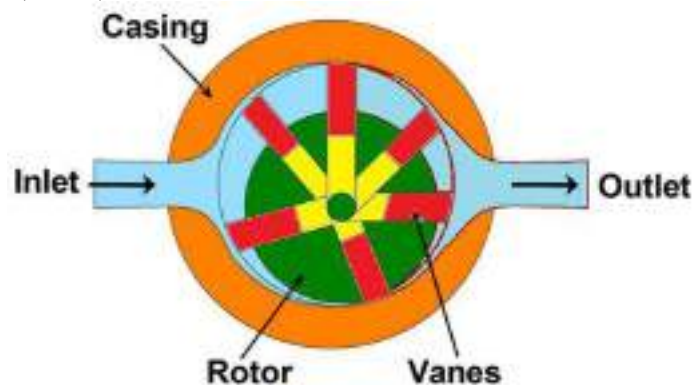
Fig. 5.3.5 Vane motor
